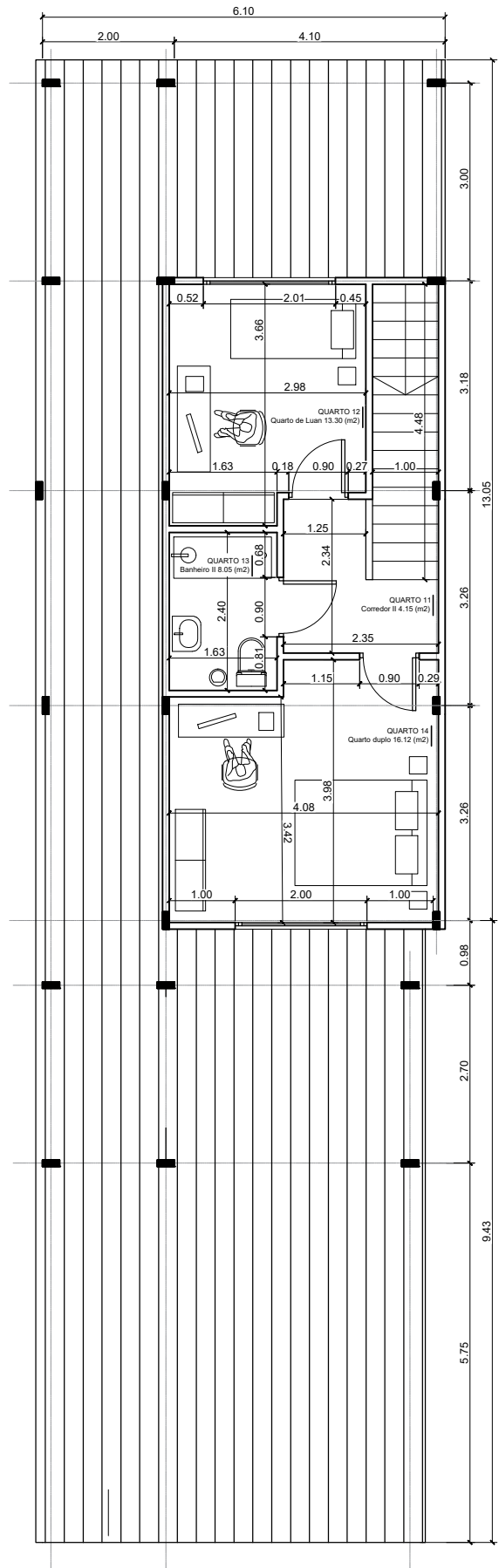
SEGUNDO ANDAR *escala 1.100
